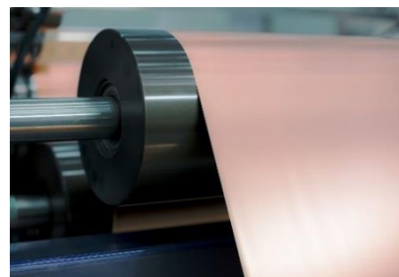
双面光电解铜箔4 \mu m~15 \mu m
